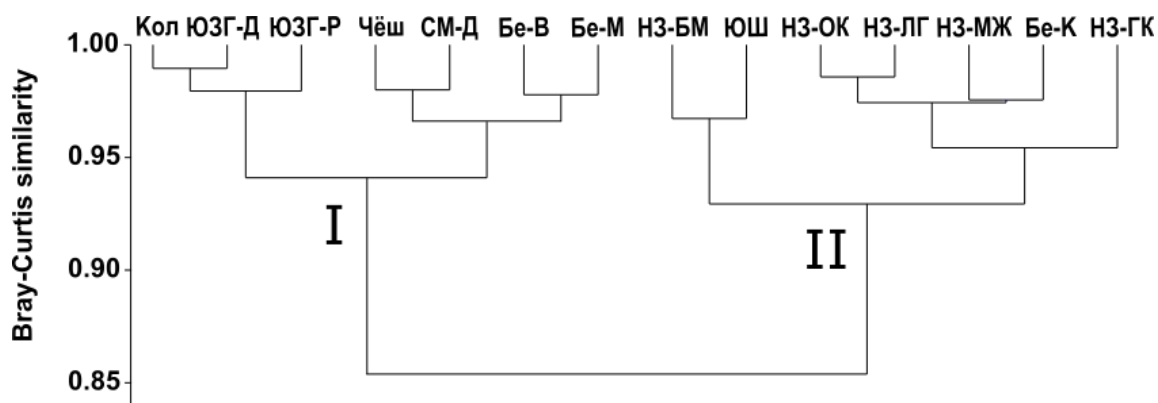
Рис. 5. Дендрограмма сходства роста новоземельских мидий морфотипа ЕМ и вида M. edulis из различных сублиторальных поселений
